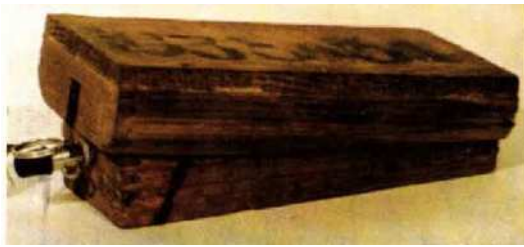
Протипіхотна міна ПМД в дерев'яному корпусі (фугасна)
